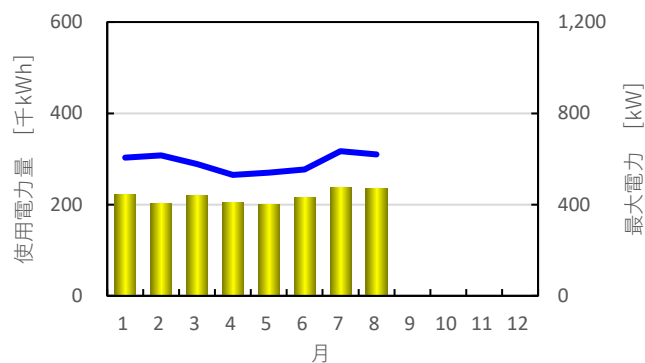
整備棟
